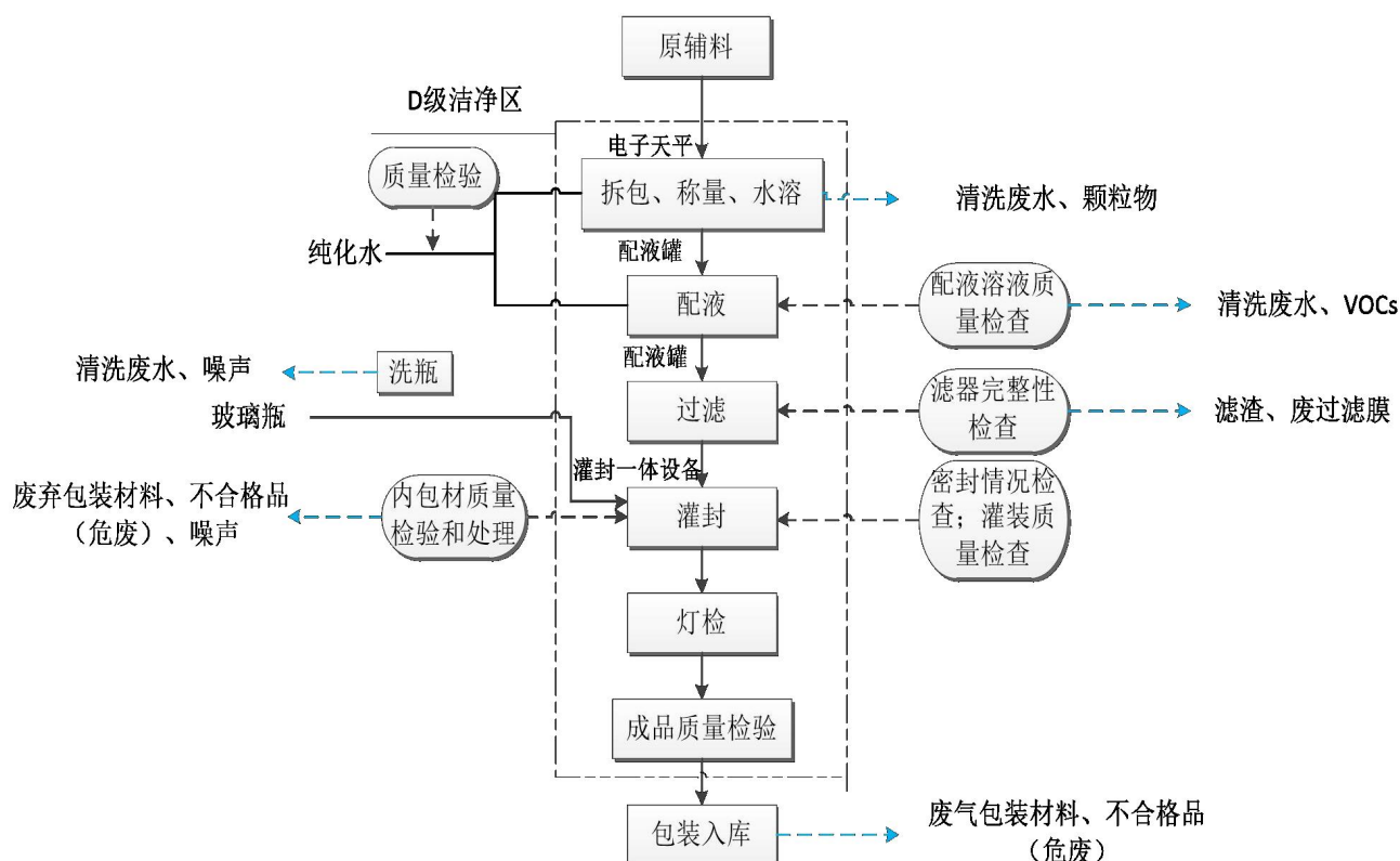
图2-2 蒙脱石混悬液生产工艺流程图
