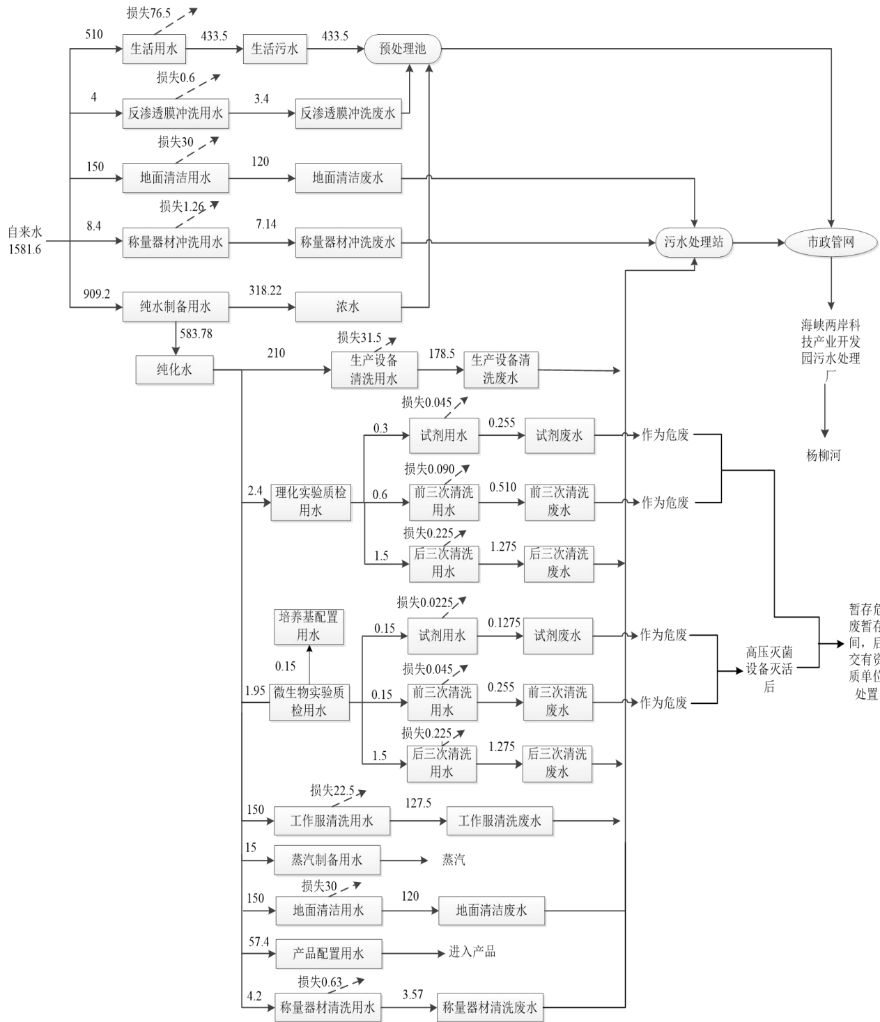
图 2-1 水平衡图单位: m³/a
