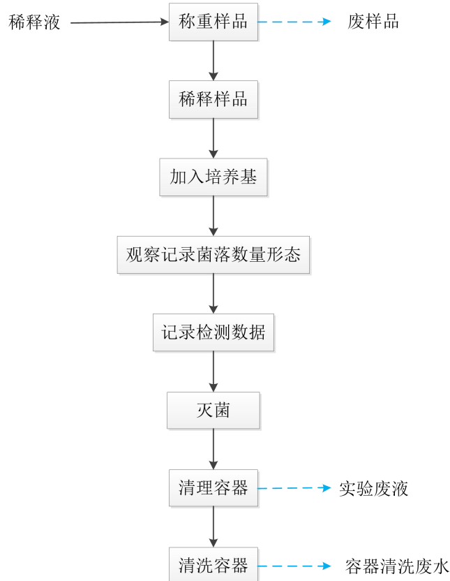
图 2-8 微生物实验工艺流程及排污节点图
