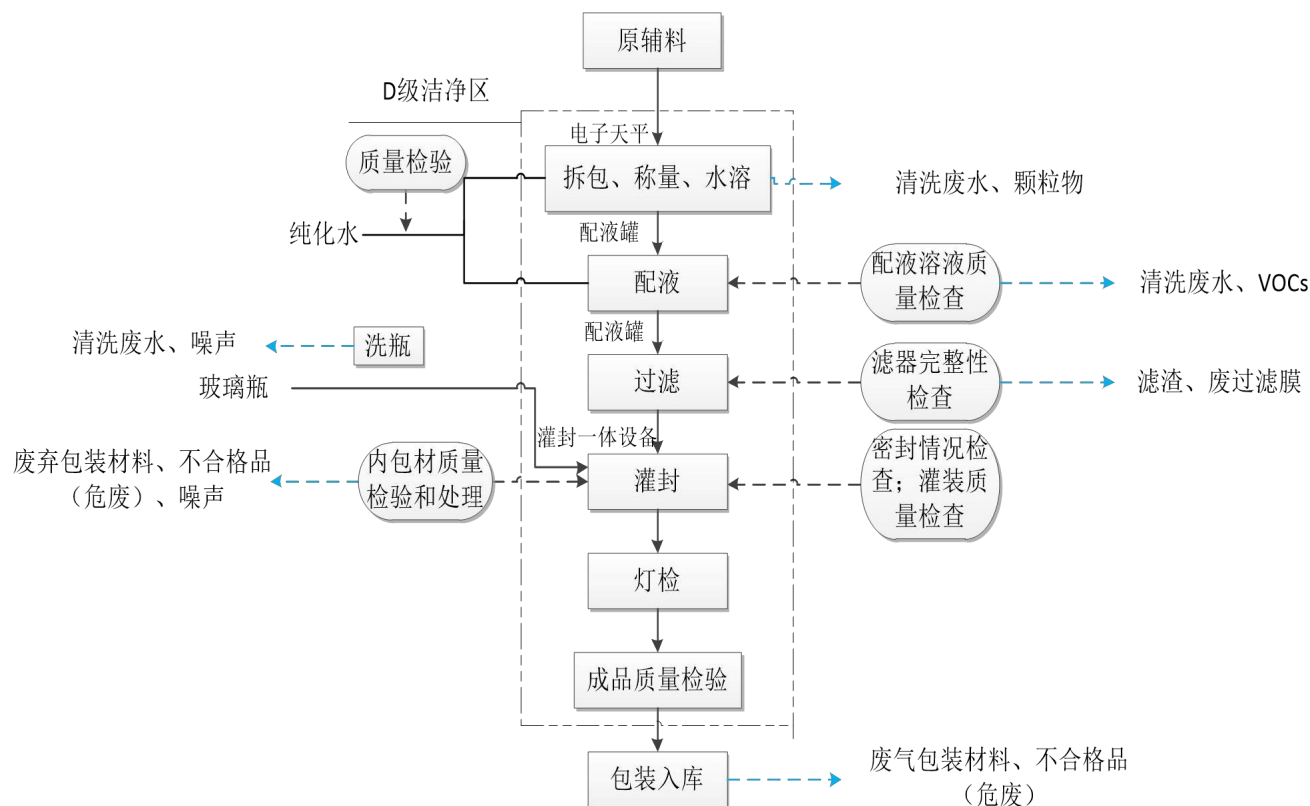
图2-3 丙戊酸钠口服溶液生产工艺流程图
