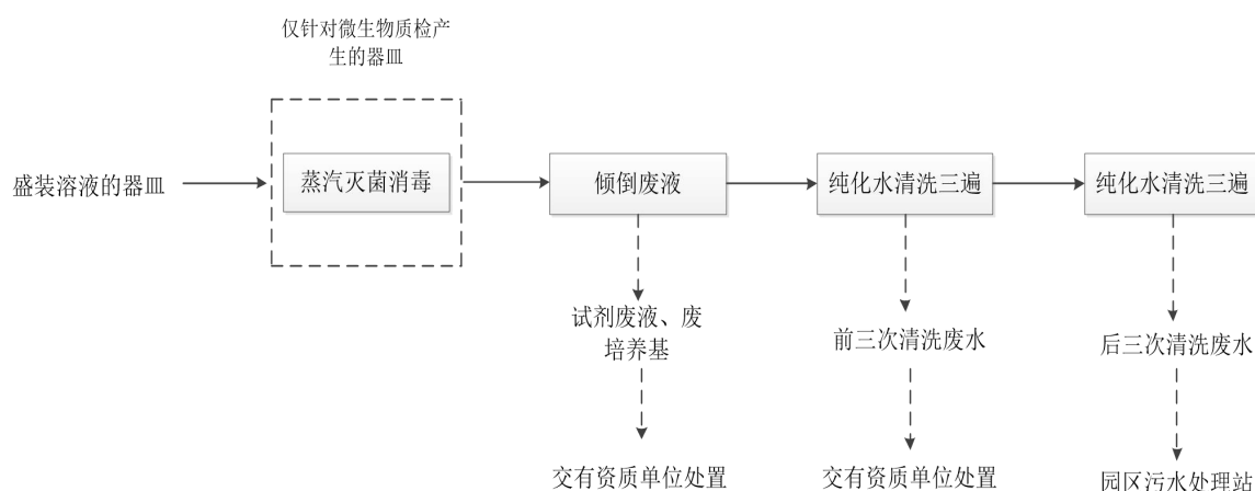
图 2-9 实验检验器皿清洗过程及产污环节分析
