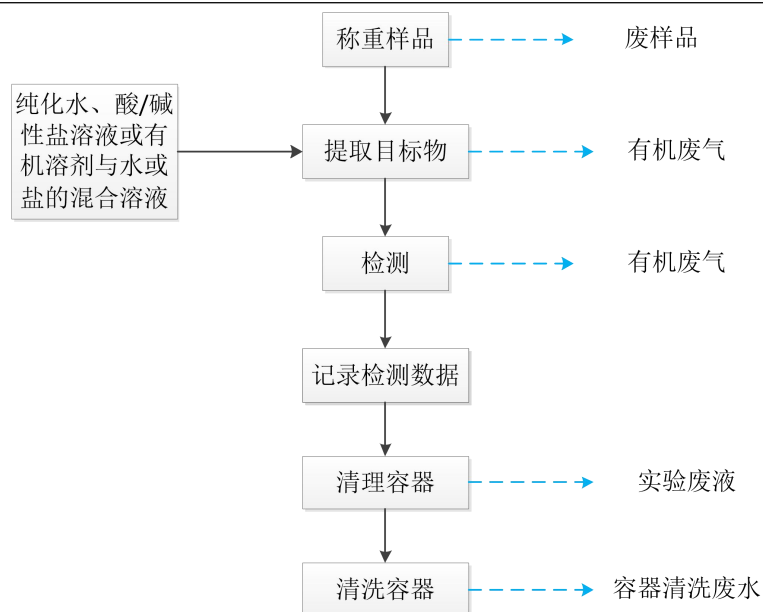
图 2-7 其他理化实验工艺流程及排污节点图
