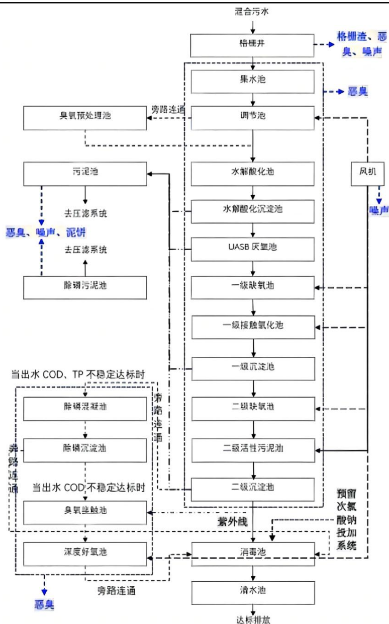
图 3-1 标准厂房园区污水处理站工艺流程示意图
