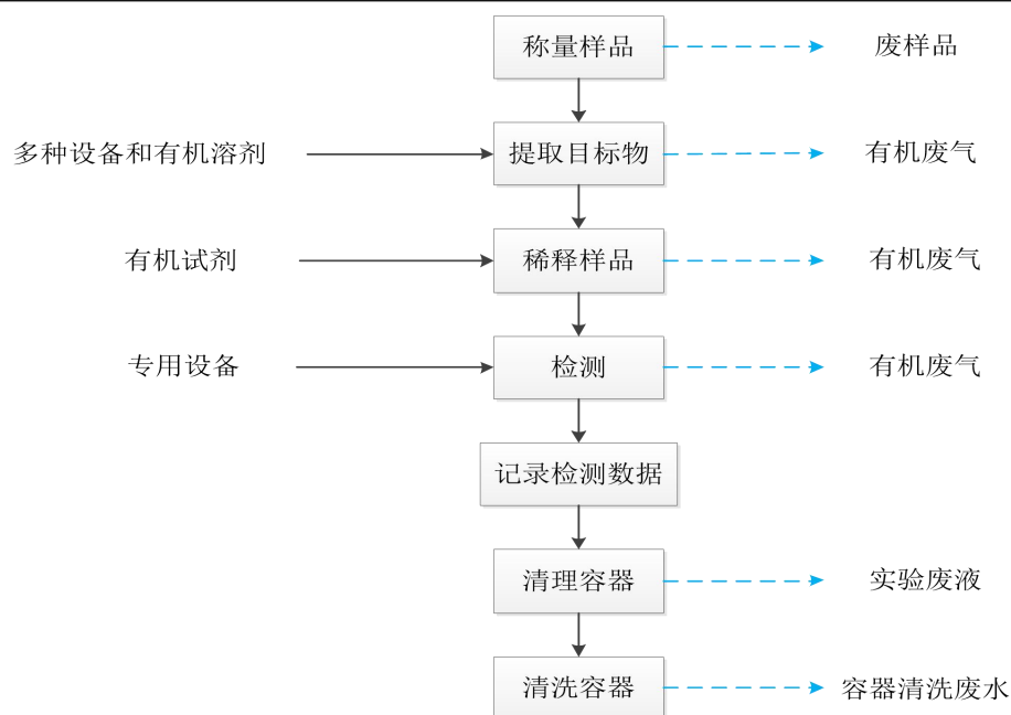
图 2-5 有机实验工艺流程及排污节点图
